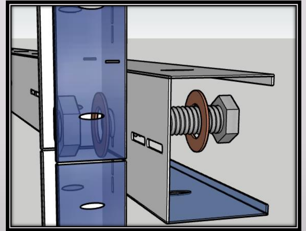
Vis , rondelle et écrou de 13
