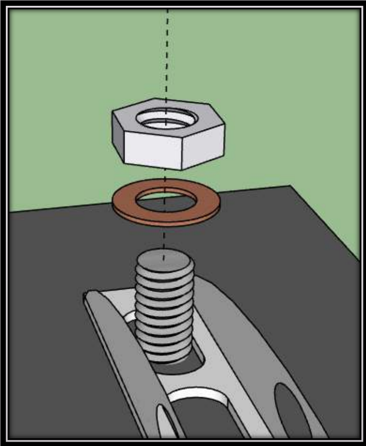
Montage jumelage avec socle
