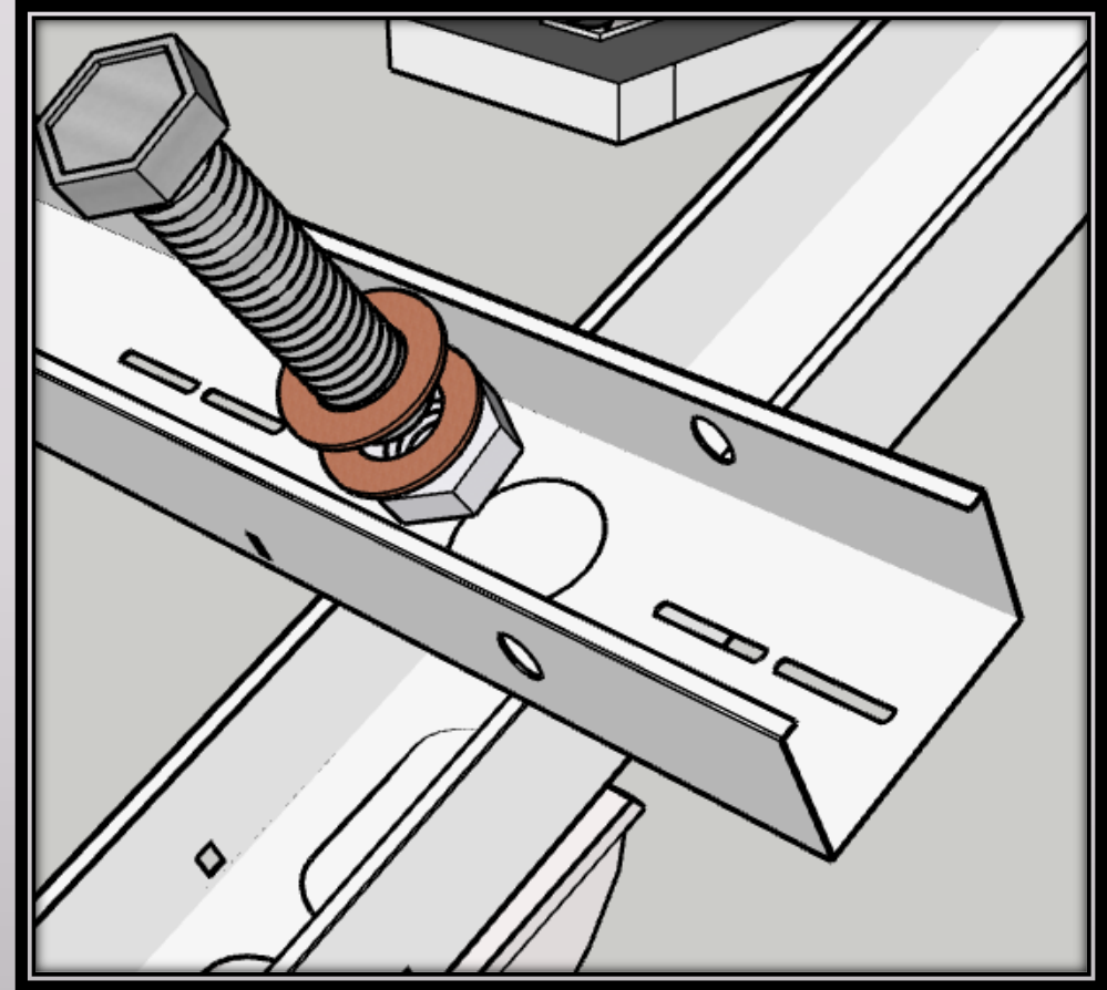
Vis , rondelle et écrou de 13
